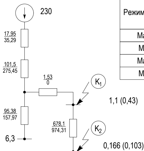
Схема замещения
